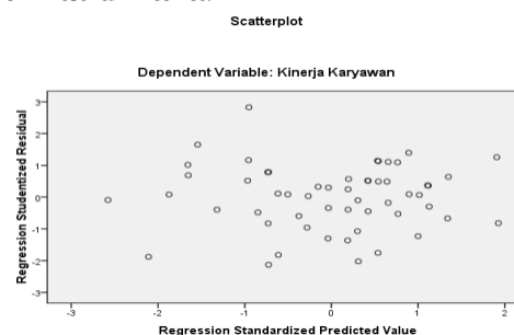
Gambar 3. Uji Heteroskedastisitas
